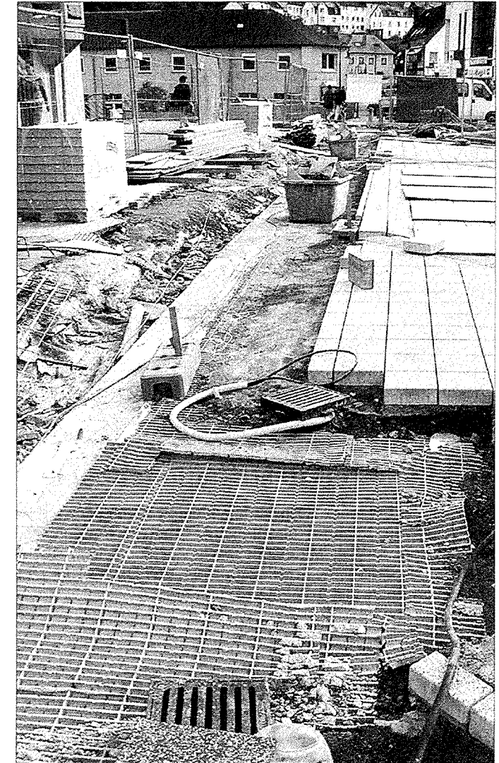
Im Bautagebuch sind Fotos zu finden, die – nach Ansicht der Bauleitung – Mängel auf der Baustelle, vor allem beschädigte Drainmatten, dokumentieren.
