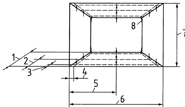
Bild 10 — Prüfung der lichten Breite eines Raumes
